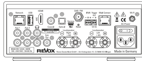
Rückansicht M300
